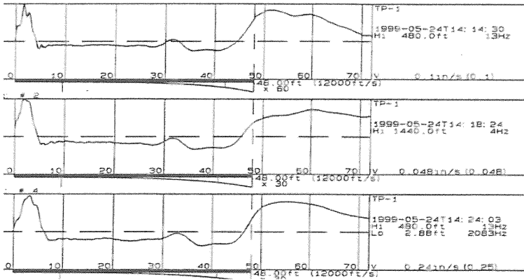
Bild 3: Schneckenbohrpfahl; Low Strain Messung mit Reflexion bei 28 ft
