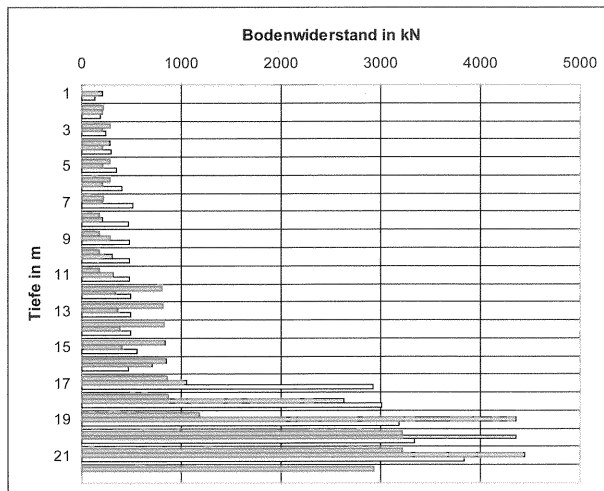
Bild 7: Dynamisch ermittelte Bodenwiderstandsverteilung von 3 Bohrpfählen
