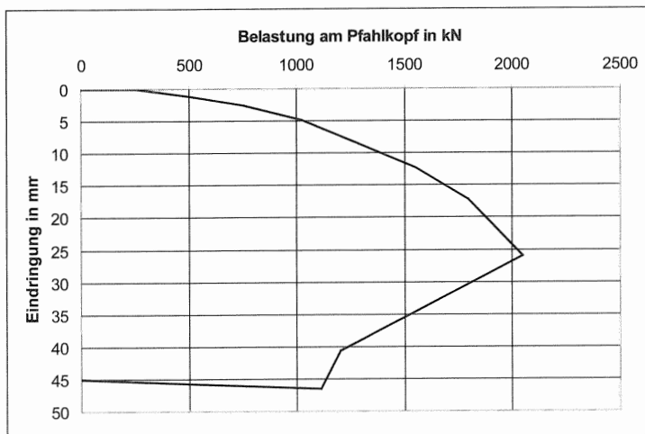
Bild 2: Last-Setzungskurve, Schneckenbohrpfahl
