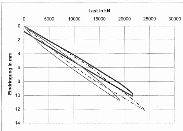
Bild 6: Dynamisch ermittelte Last-Setzungskurven von 3 Bohrpfählen
