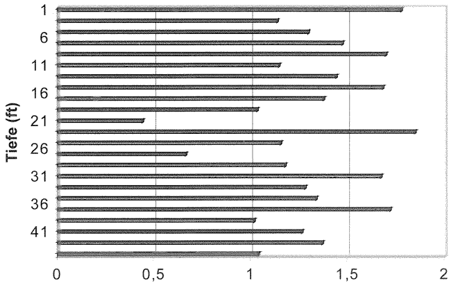
Bild 4: Schneckenbohrpfahl: Verhältnis Messvolumen / Soll-Volumen
